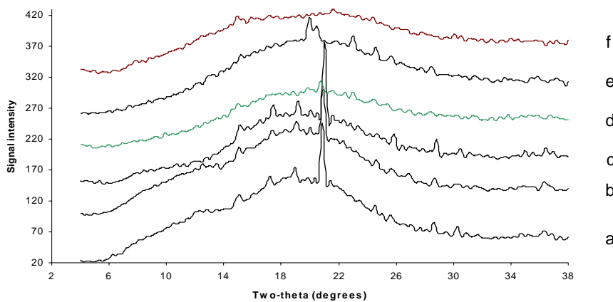
نمودار ۴. الگوی دیفرکسیون X-ray نمونه‌های انجیر تیمار یافته با ۴۰٪ گلوکز سیراب به تعادل رسیده در فعالیت آبی‌های (a: ۰/۱۱۲، b: ۰/۲۲۷، c: ۰/۳۸۲، d: ۰/۶۴۳، e: ۰/۷۴۳، f: ۰/۸۴۳) در دمای ۲۵ °C
