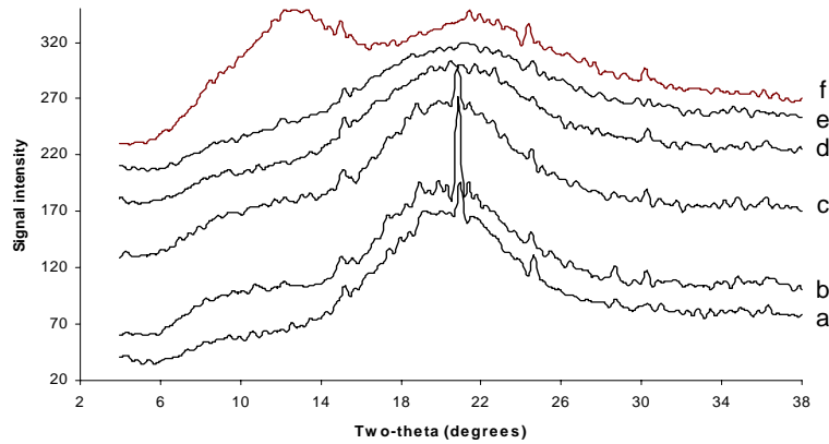
نمودار ۳. الگوی دیفرکسیون X-ray نمونه‌های انجیر تیمار یافته با ۴۰٪ گلیسرول به تعادل رسیده در فعالیت آبی‌های مختلف (a: ۰/۱۱۲، b: ۰/۲۲۷، c: ۰/۳۸۲، d: ۰/۶۴۳، e: ۰/۷۴۳، f: ۰/۸۴۳) در دمای ۲۵ °C
