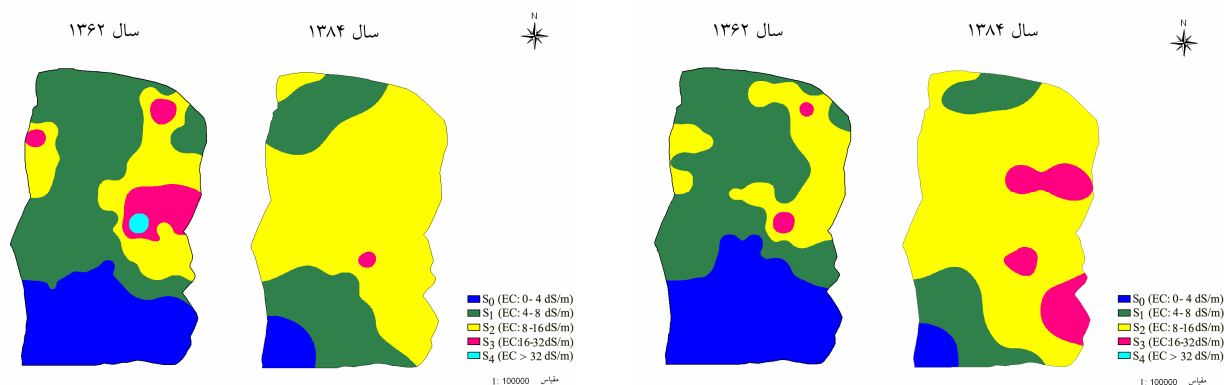
شکل ۳. نقشه شوری در عمق ۰-۵۰ سانتی متری
