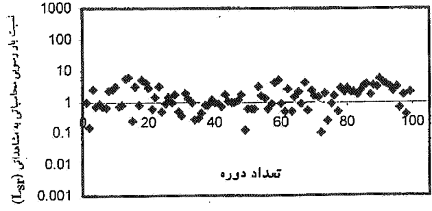
نمودار ۱-۷. روش انگلاند و هانسن، رودخانه دز
