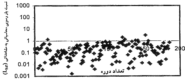
نمودار ۲-۷. روش انگلاند و هانسن، رودخانه کرخه
