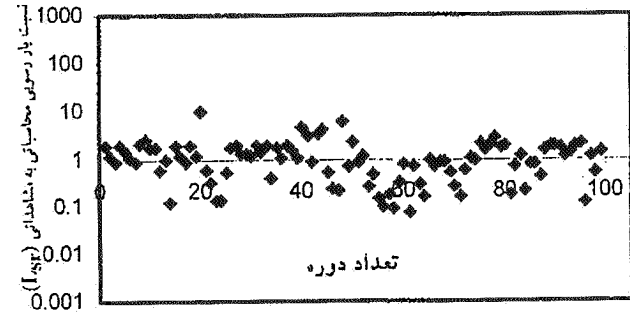
نمودار ۳-۷. روش انگلاند و هانسن، رودخانه کارون
