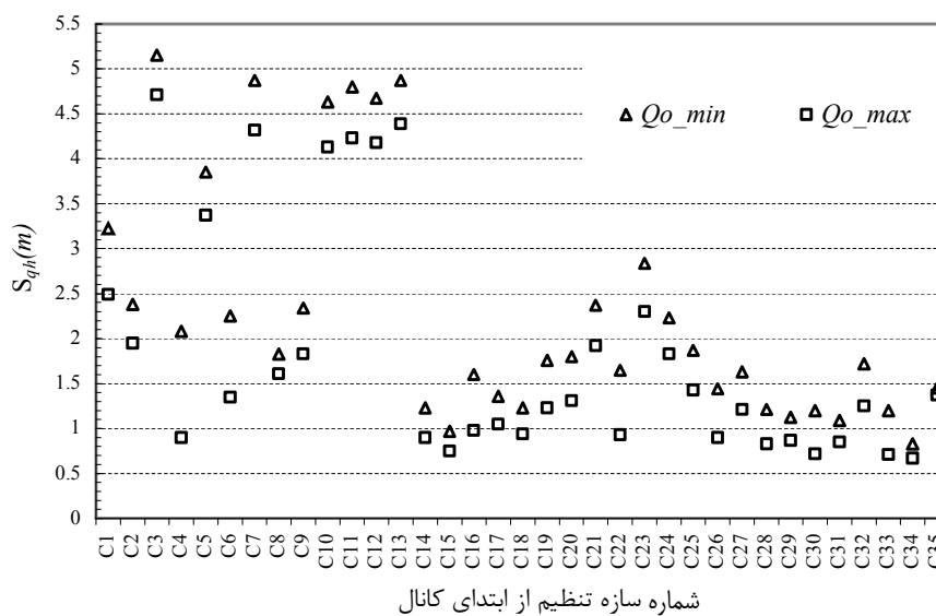
شکل ۴. مقادیر کمی شاخص‌های حساسیت عمق بده سازه‌های تنظیم کانال وادودارا
