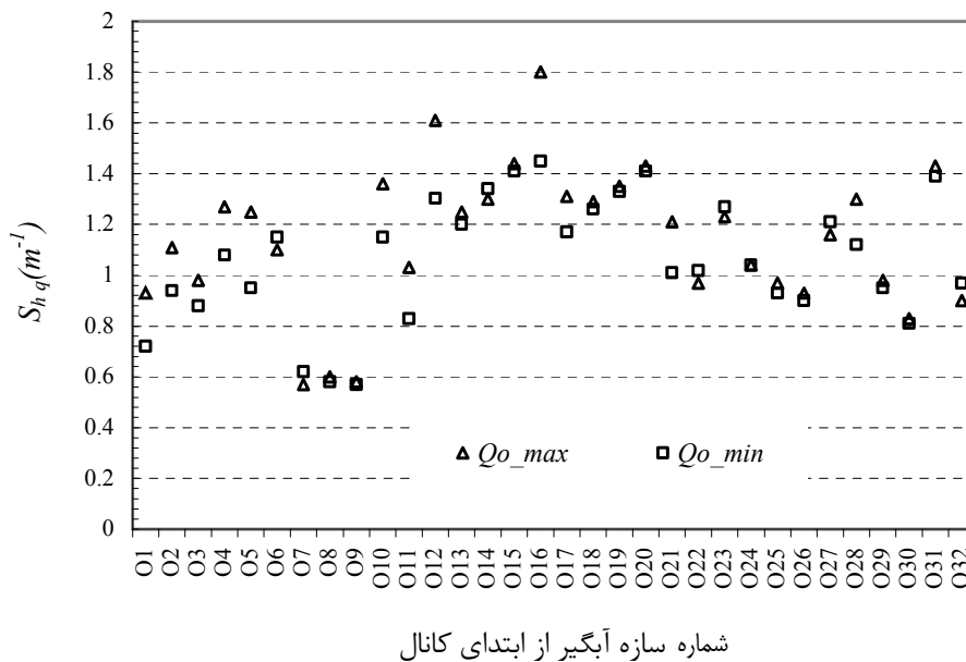
شکل ۳. مقادیر کمی حساسیت هیدرولیکی بده به عمق سازه‌های آبگیر کانال وادودارا
