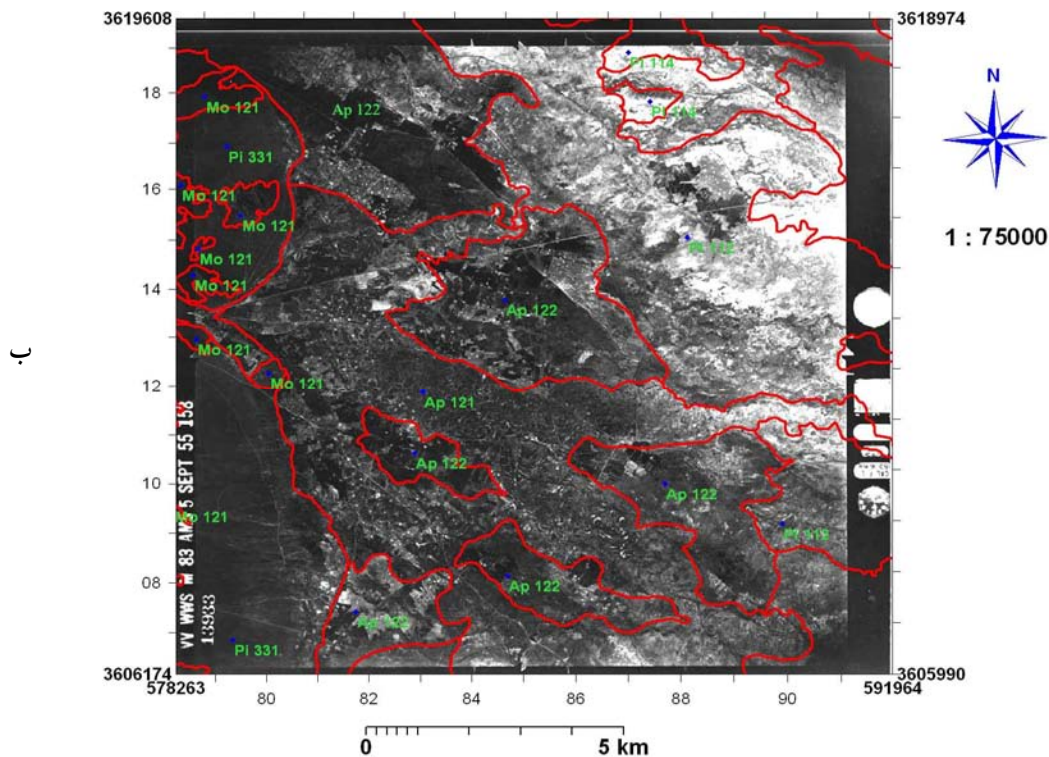
شکل ۲. الف) منابع اراضی متفاوت حاصل فرایندهای هیدرولوژی و زمین ریخت ساختی مختلف در پلاهای سکزی. رسوبات بادی روی پلاهای (W/P)، بادی روی لاگونی (W/L)، بادی روی پلاهای روی رودخانه‌ای (W/P/R)، شماره‌های داخل متن تصویر عبارت از مسیرهای اول تا سوم رودخانه زاینده رود در دوران چهارم زمین شناسی می باشند. ب) آبرفت‌های قدیمی رودخانه زاینده رود در مسیرهای یک (Ap 122) و دو (Ap 121) نشان داده شده در بالا
