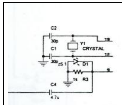
شکل ۶. مدار ساعت و راه‌انداز میکروکنترلر
