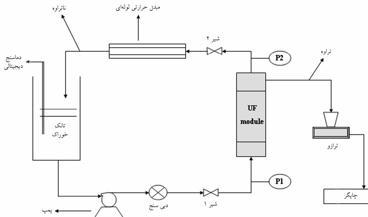
شکل ۲. شماتیک کلی، واحد یا یلوتی، UF
