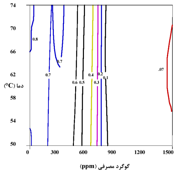
شکل ۲. خطوط هم تراز رنگ برای نمونه‌های تهیه شده به روش BSD (بیشترین تأثیرگذاری گوگرد و در نتیجه تراکم خطوط هم رنگ در محدوده ۴۰۰ تا ۸۰۰ ppm دیده می‌شود).
