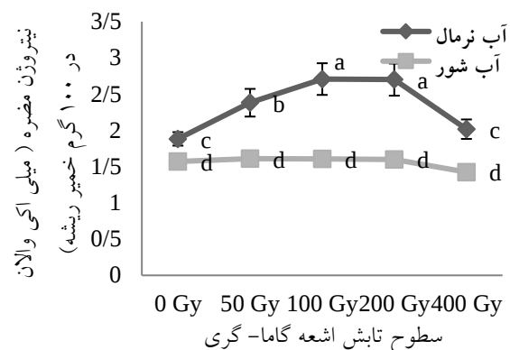
شکل ۱۰. مقایسه تغییرات غلظت نیترژن مضره تحت اثر برهم‌كنش تنش شوری و سطوح مختلف تابش اشعه گاما. میانگین‌های دارای حروف مشابه طبق آزمون دانكن در سطح احتمال ۱٪ اختلاف معنی‌داری با یکدیگر ندارند.
