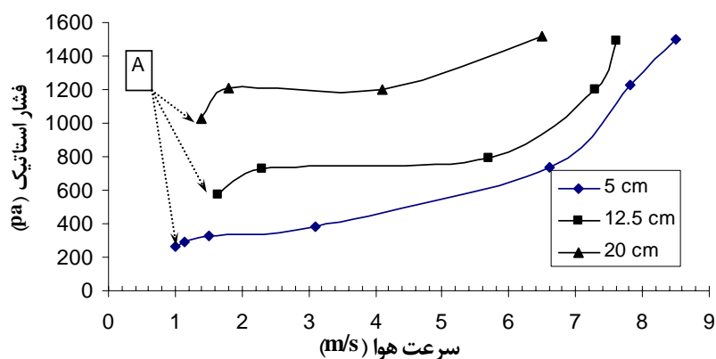
شکل ۲. منحنی مشخصه افت فشار- سرعت هوا برای شرایط بستر سیال در عمق های ۵ cm، ۱۲/۵ cm و ۲۰ cm (نقطه A= نقطه حداقل سیال سازی)
