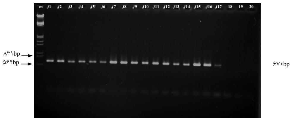
شکل ۴. تکثیر باند ۶۷۰ جفت بازی توسط جفت آغازگر OPAFjav / OPARjav در جمعیت‌های مختلف گونه M. javanica (J1-)
