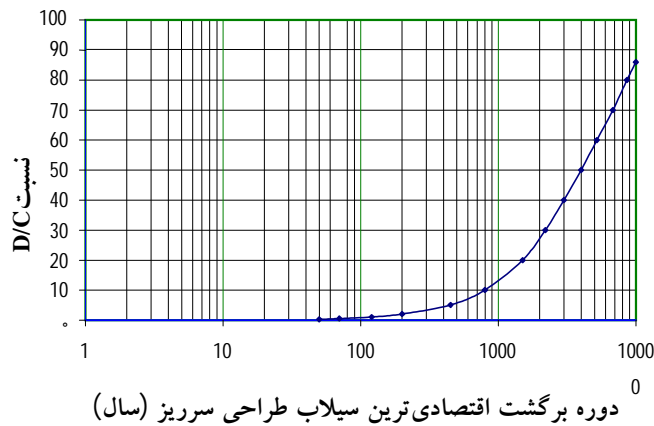
شکل ۱. منحنی واحد برای انتخاب اقتصادی‌ترین سیلاب طراحی سرریز (۷)
