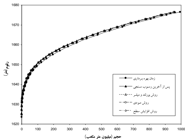
شکل ۷. منحنی‌های ارتفاع - حجم اولیه، ثانویه و پیش‌بینی شده برای سد دروزن
