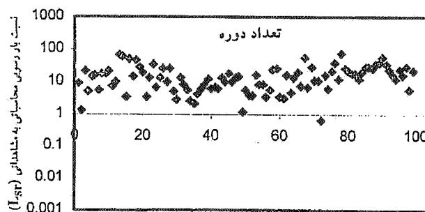
نمودار ۶-۱. روش وایف، رودخانه دز
