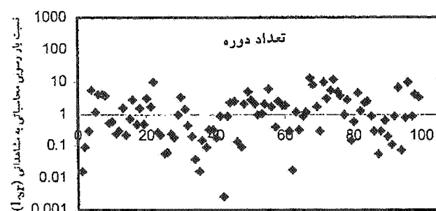
نمودار ۲-۴. روش توفالتي، رودخانه کرخه
