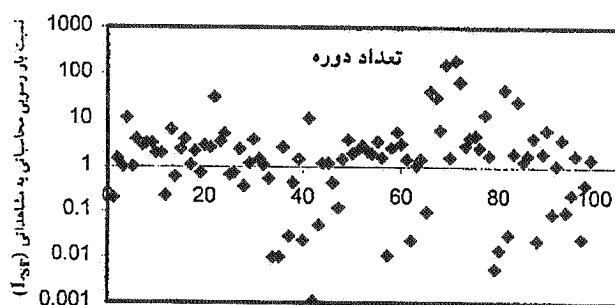
نمودار ۶-۲. روش وایف، رودخانه کرخه
