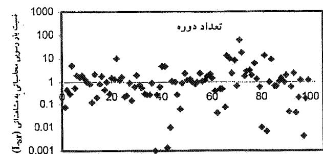
نمودار ۲-۸. روش یانگ، رودخانه کرخه
