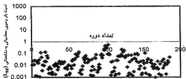
نمودار ۴-۲. روش بگنولد، رودخانه مارون
