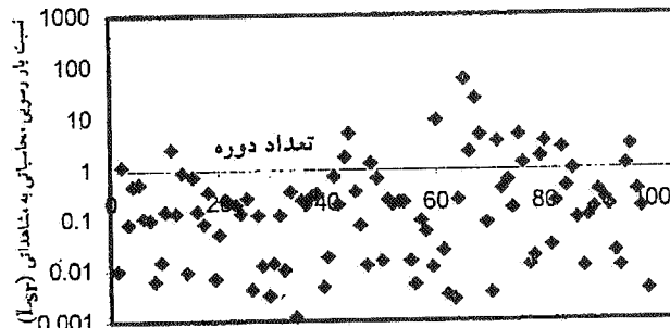
نمودار ۱-۳. روش انیشتین، رودخانه کارون
