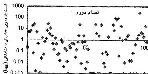
نمودار ۵-۱. روش وان‌ریجن، رودخانه دز
