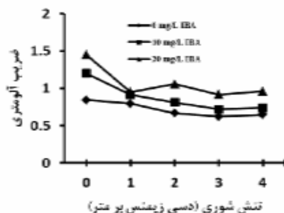
شکل ۵. برهمکنش تنش شوری و ایندول بوتیریک اسید بر ضرب الومتری لوبیا
