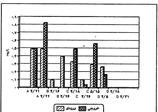
نمودار ۱۳. تغییرات غلظت NO ۳ در آب ورودی و خروجی مزارع
