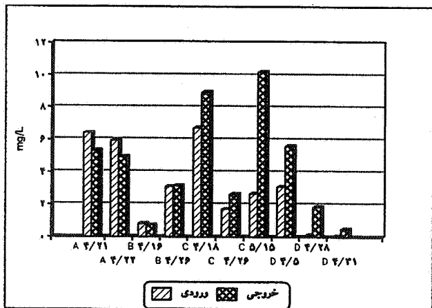
نمودار ۱۴. تغییرات غلظت NH ۴ در آب ورودی و خروجی مزارع
