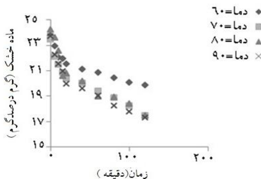
شکل ۱. سینتیک تغییرات ماده خشک طی آنزیم ببری در دماهای مختلف
