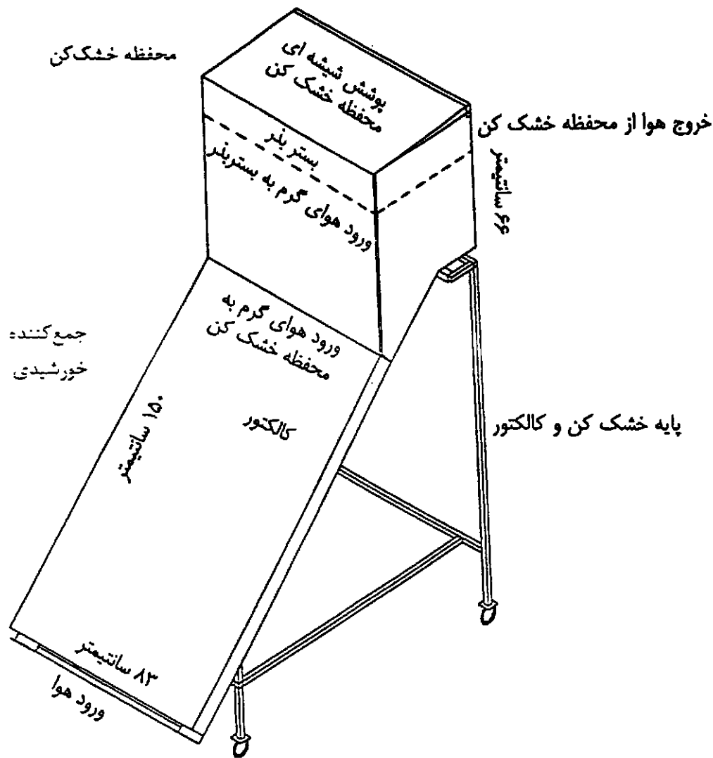
شکل ۱. تصویر شماتیک خشک کن خورشیدی
