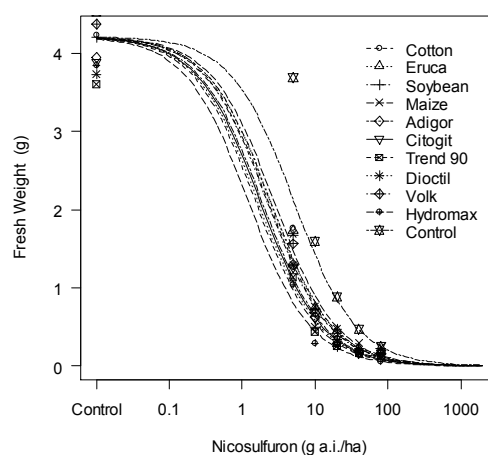
شکل ۲. منحنی دز- پاسخ تاج خروس ریشه قرمز به مقادیر مختلف علف کش نیکوسولفورون در سطوح مواد افزودنی مختلف
