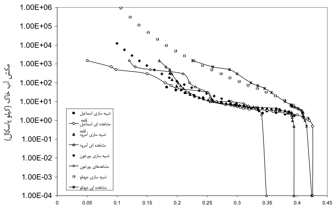
شکل ۲. مقادیر اندازه گیری و شبه سازی شده منحنی مشخصه آب خاک در بافت های شنی، لوم رسی شنی، لومی و لوم رسی لایی (به ترتیب در سری های اسماعیل قلمه، آمروود آغاچ، یورغون آباد و جهتلو)
