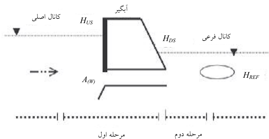
شکل ۳. وضعیت جریان در سازه آبگیر
