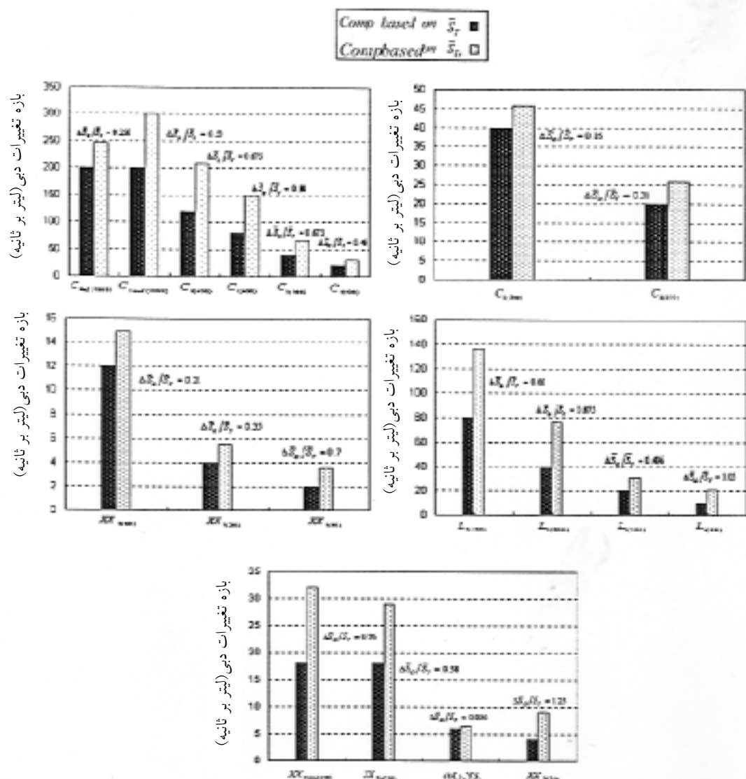
شکل ۸. مقایسه بازه تغییرات دبی شرایط تئوری و بهره‌برداری مدول‌های مورد بررسی
