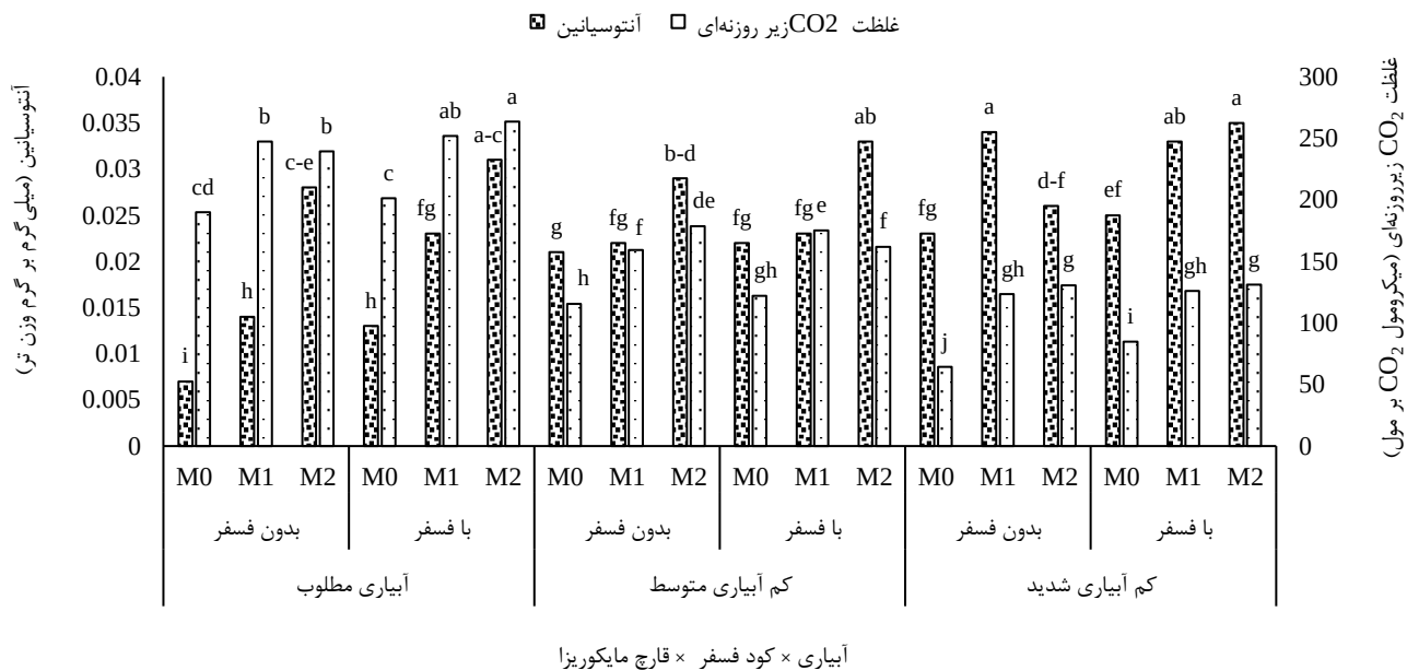
شکل ۴. مقایسه میانگین برهم‌کنش سه‌گانه آبزیایی در کود فسفر در قارچ مایکوریزا بر محتوای آنتوسیانین و غلظت CO 2 زیر ریشه‌ای برگ خیار تلخ
