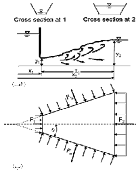
شکل ۱. نمای کلی جهش هیدرولیکی در حوضچه دوزنقه‌ای واگرا
