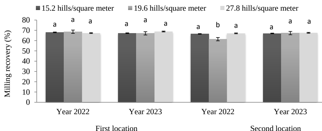
شکل ۴. راندمان تبدیل (درصد) تحت اثر متقابل مکان × سال × تراکم گیاهی. میانگین‌هایی که با حرف یکسانی مشخص شده‌اند، بر اساس آزمون توکی در سطح احتمال پنج درصد تفاوت معنی‌داری ندارند.
