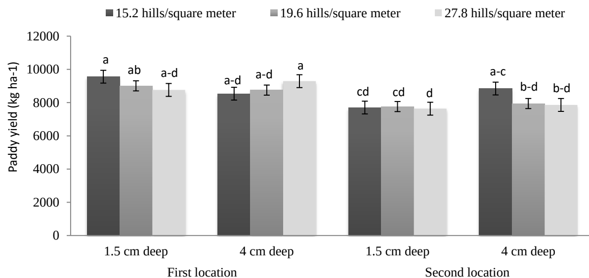
شکل ۳. عملکرد شلتوک (کیلوگرم در هکتار) تحت اثر متقابل مکان × عمق کاشت × تراکم گیاهی. میانگین‌هایی که با حرف یکسانی مشخص شده‌اند، بر اساس آزمون توکی در سطح احتمال پنج درصد تفاوت معنی‌داری ندارند.
