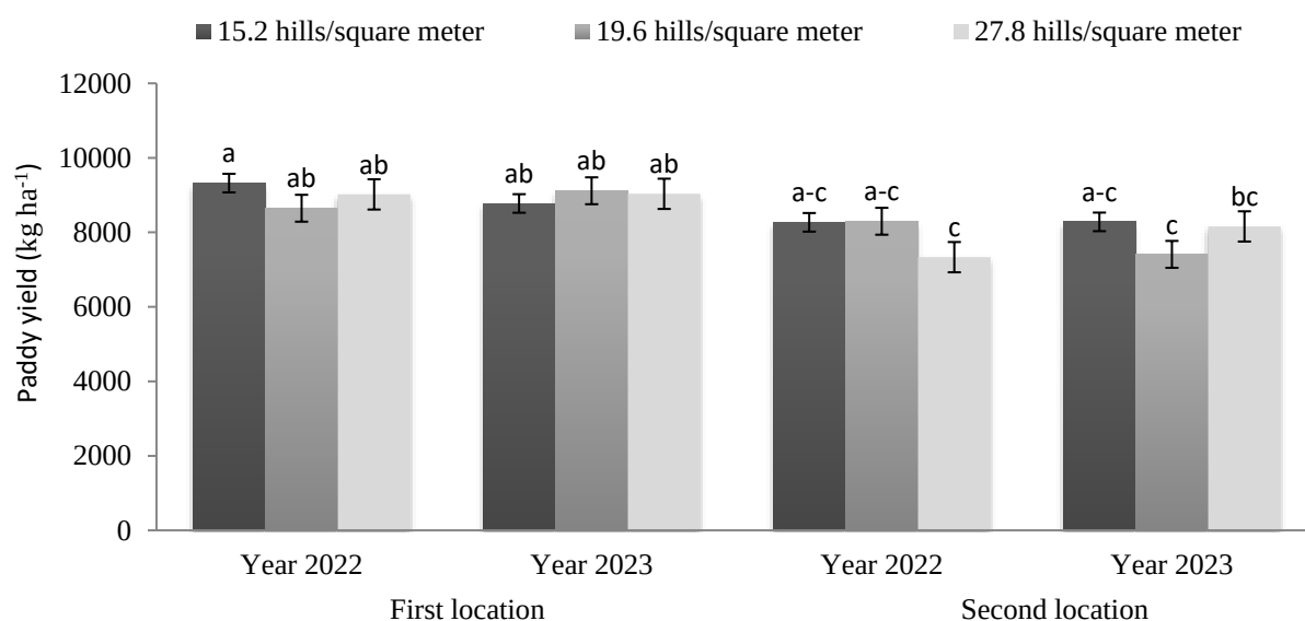
شکل ۲. عملکرد شلتوک (کیلوگرم در هکتار) تحت اثر متقابل مکان × سال × تراکم گیاهی. میانگین‌هایی که با حرف یکسانی مشخص شده‌اند، بر اساس آزمون توکی در سطح احتمال پنج درصد تفاوت معنی‌داری ندارند
