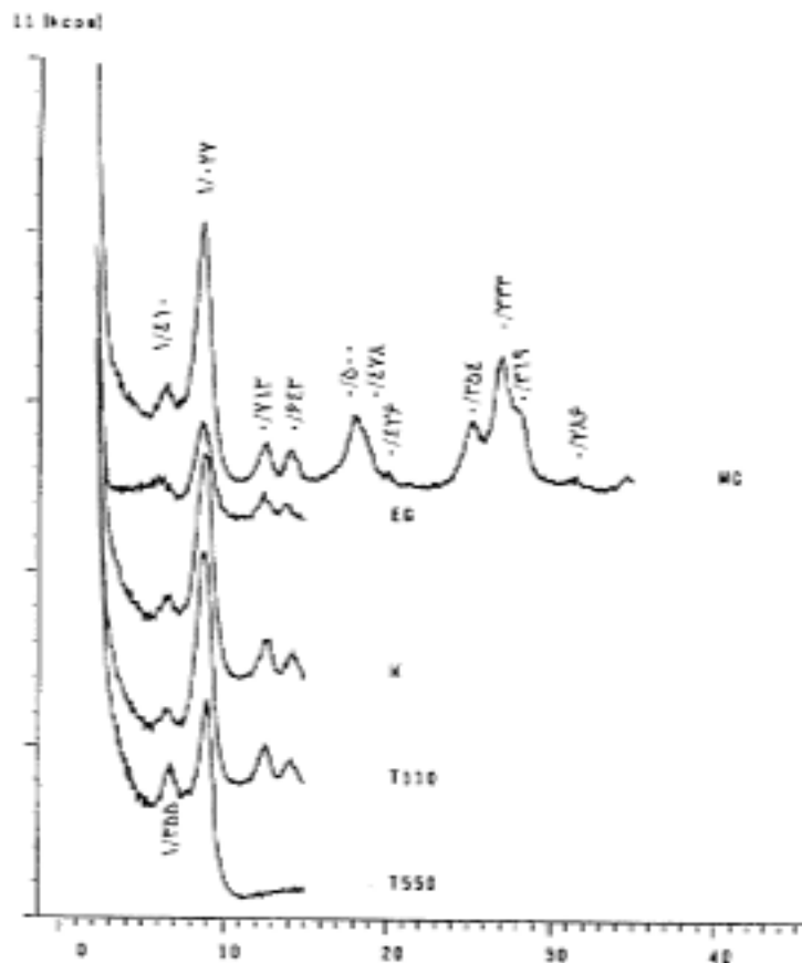
شکل ۲. پراش نگاشت‌های پرتو X ذرات رس ریز افق Byk نیم‌رخ اول مخروط افکنه پایکوهی (A۱)
