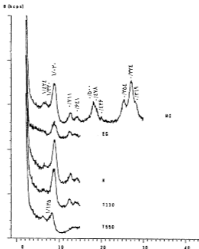
شکل ۷. پراش نگاشت‌های پوتو X ذرات رسی ریز افق 2Bzy نیمرخ اول تراس قدیمی رودخانه (T۱)
