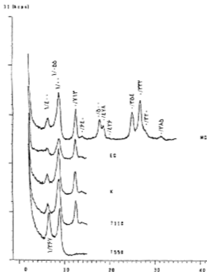
شکل ۳. پراش نگاشت‌های پرتو X ذرات رس درشت افق Byk نیم‌رخ اول مخروط افکنه پایکوهی (A۱)
