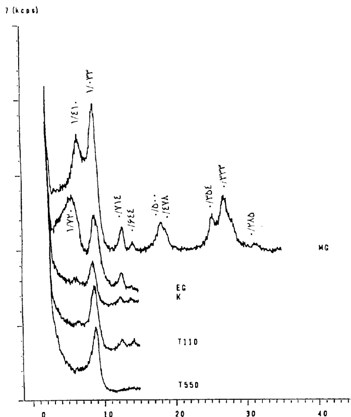
شکل ۸. پراش نگاشت‌های پرتو X ذرات رس ریز افق 2Bz1 نیم‌رخ دوم ترانس قدیمی رودخانه (T۲)
