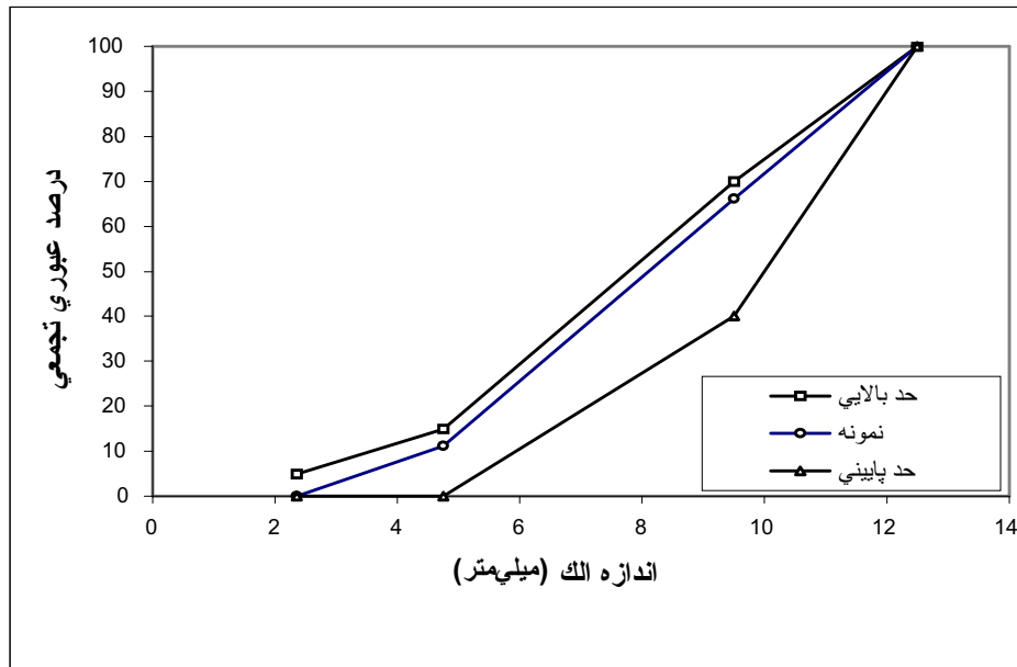
شکل ۱. منحنی دانه‌بندی مصالح درشت‌دانه
