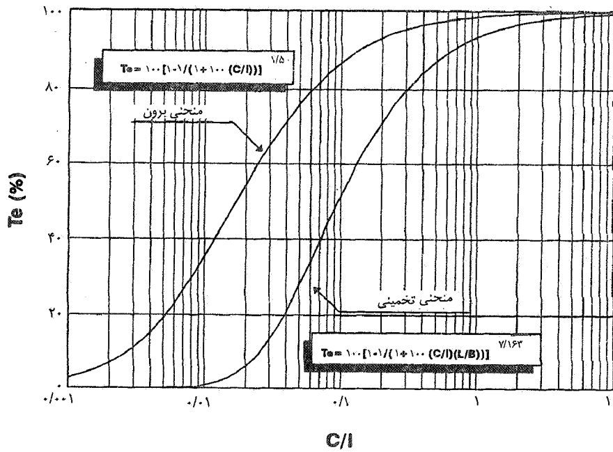
شکل ۳- مقایسه منحنی های به دست آمده از معادله (A) و منحنی برون
