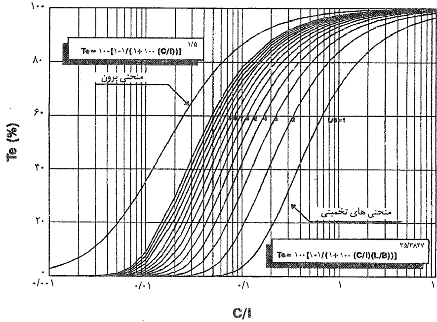
شکل ۲- مقایسه منحنی های به دست آمده از معادله (V) و منحنی برون
