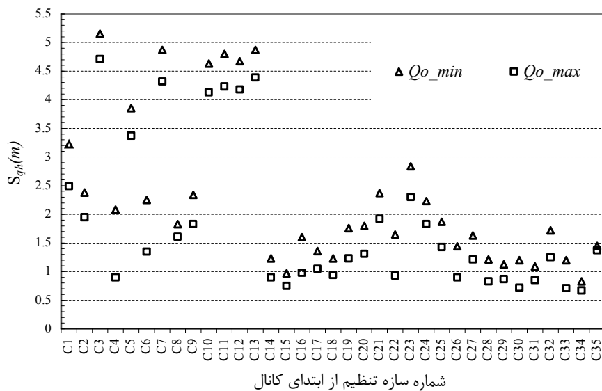
شکل ۴. مقادیر کمی شاخص‌های حساسیت عمق بده سازه‌های تنظیم کانال وادودارا
