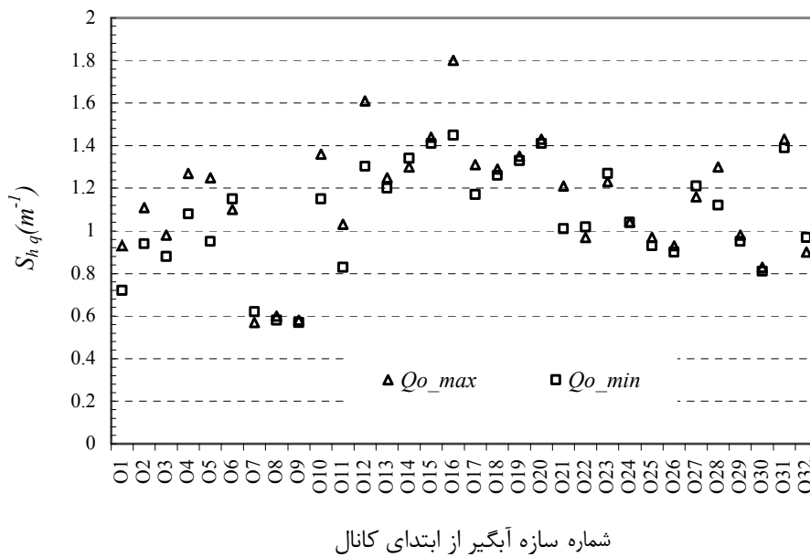
شکل ۳. مقادیر کمی حساسیت هیدرولیکی بده به عمق سازه‌های آبگیر کانال وادودارا
