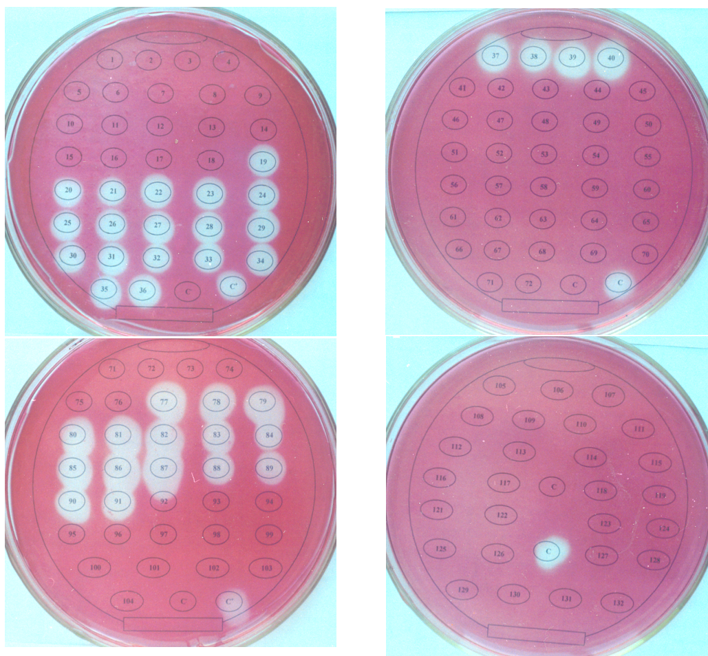
شکل ۳. بررسی فعالیت آنزیم پلی گالاتوروناز به روش test plate :
