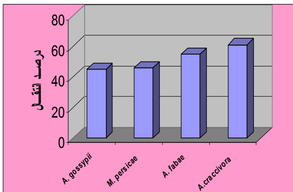
شکل ۸. نمودار میانگین درصد انتقال سه ویروس شته زاد توسط چهار گونه شته
