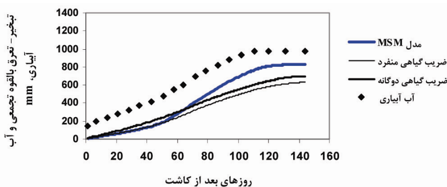
شکل ۹. مقایسه مقادیر تبخیر-تعرق بالقوه تجمعی پیش‌بینی شده با استفاده از مدل MSM، ضرایب گیاهی دوگانه و
