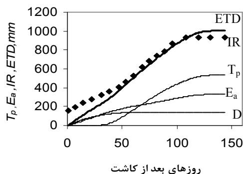
شکل ۲. مقادیر پیش‌بینی شده نفوذ عمقی (D)، تبخیر ( E_a )، تعرق بالقوه ( T_p )، مجموع تبخیر، تعرق بالقوه و نفوذ عمقی (ETD) توسط مدل MSM و مقادیر اندازه‌گیری شده آب آبیاری و بارندگی (IR) در سال ۱۳۸۲
