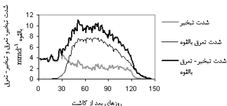
شکل ۳. شدت تبخیر، تعرق و تبخیر-تعرق بالقوه روزانه پیش‌بینی شده توسط مدل MSM در روزهای مختلف بعد از کاشت در سال ۱۳۸۲
