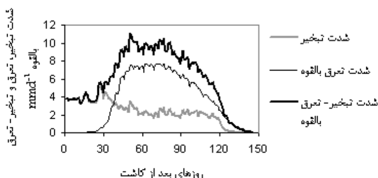
شکل ۳. شدة تبخیر، تعرق و تبخیر-تعرق بالقوه روزانه پیش‌بینی شده توسط مدل MSM
