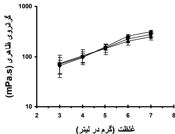
شکل ۵. نمایش تاثیر غلظت روی گرانیوی ظاهری محلول پودر ثعلب در پ هاش ۷ و دمای ۲۵ درجه سانتی گراد در سرعت های چرخشی مختلف (◆، ۷۵؛ ■، ۱۰۰؛ ▲، ۱۳۵).
