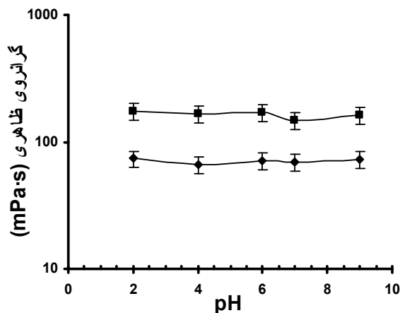
شکل ۶. نمایش تاثیر پ هاش روی گرانیوی ظاهری محلول پودر ثعلب در پ هاش ۷ و دمای ۲۵ درجه سانتی گراد در دو غلظت مختلف (◆، ۳؛ ■، ۵ گرم در لیتر) و سرعت چرخشی ثابت ۱۰۰ دور بر دقیقه.
