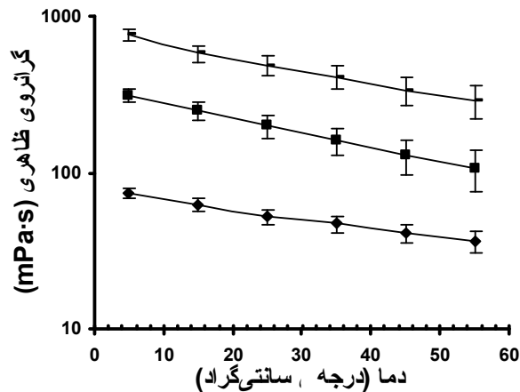
شکل ۴. نمایش تاثیر دما روی گرانیوی ظاهری محلول پودر ثعلب در پ هاش ۷ و دمای ۲۵ درجه سانتی گراد در غلظت های مختلف (◆، ۳؛ ■، ۵؛ ●، ۷ گرم در لیتر) و سرعت چرخشی ثابت ۵۰ دور بر دقیقه.
