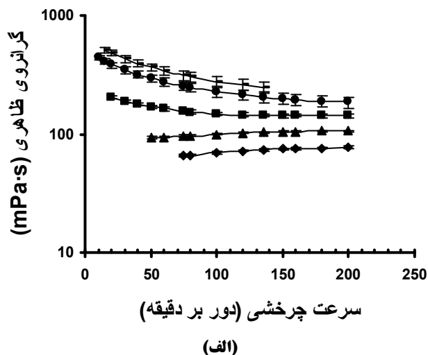
شکل ۲. نمایش رفتار جریان محلول‌های پودر ثعلب در غلظت‌های مختلف (۷، ۶، ۵، ۴، ۳، ۲ گرم در لیتر) در دمای ۲۵ درجه سانتی‌گراد و پ هاش ۷ (الف) سرعت چرخشی در مقابل گرانیوی ظاهری (ب) سرعت برشی در مقابل گرانیوی ظاهری.
