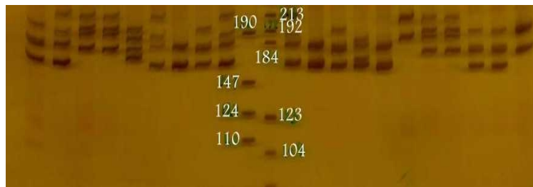
شکل ۱. الگوی باندها برای جایگاه MCMA2
