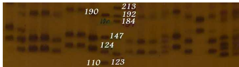
شکل ۲. الگوی باندها برای جایگاه BMS460
