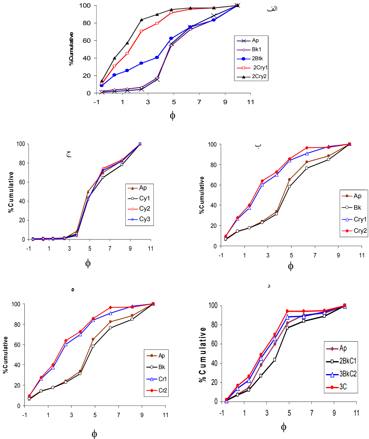
شکل ۳. منحنی تجمعی توزیع اندازه ذرات در خاک‌های مورد مطالعه
