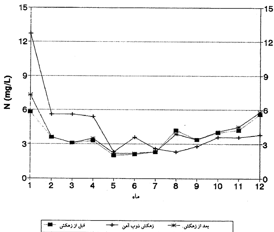
شکل ۴. تغییرات ماهیانه غلظت ازت معدنی در زه آب زهکشی ذوب آهن و آب زاینده رود در سال ۱۳۷۷
