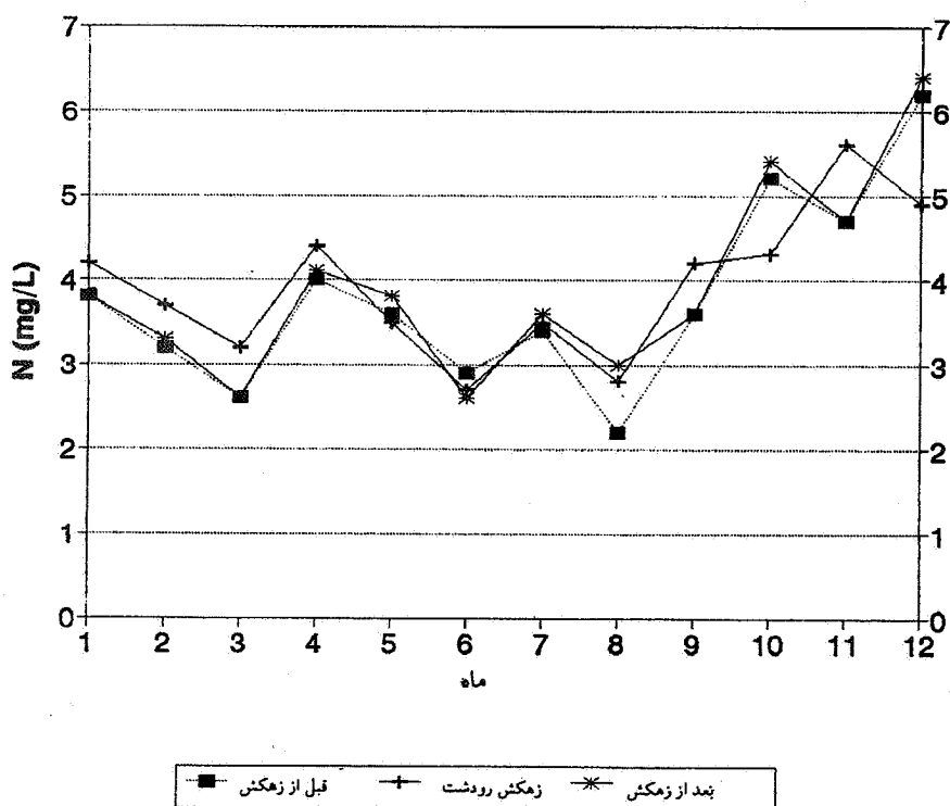
شکل ۵. تغییرات ماهیانه غلظت ازت معدنی در زه آب زهکشی رودشت و آب زاینده رود در سال ۱۳۷۷
