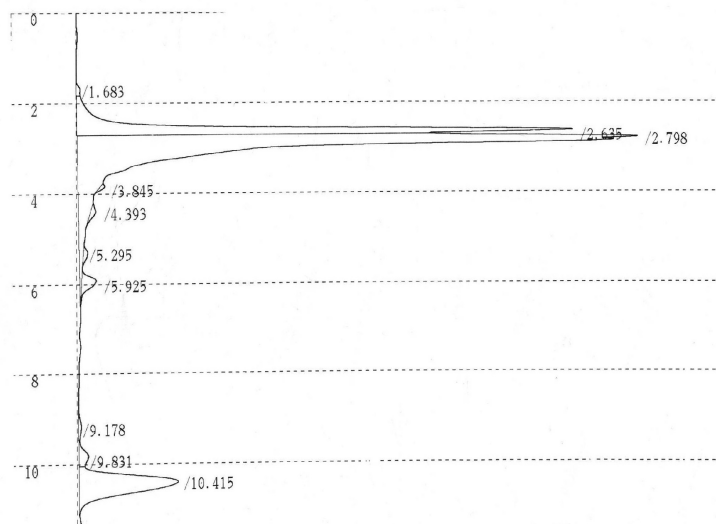
شکل ۲. کروماتوگرام HPLC عصاره ریشه شیرین بیان، شرایط کروماتوگرافی: ستون (RP-C 18 (150 × 4.6 mm)، دمای آون °C ۴۰، آشکار ساز UV (طول موج ۲۵۴ nm)، فاز متحرک: متانول-آب-اسید استیک (۷۵V/V/V : ۲۴ : ۱)، سرعت جریان ۱ میلی لیتر در دقیقه
