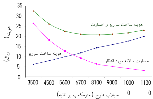
شکل ۴. برآورد هزینه‌های ساخت سرریز و خسارت مورد انتظار متناظر با گزینه‌های مختلف طراحی سرریز سد پیشین (روش مهندسی عمران)
