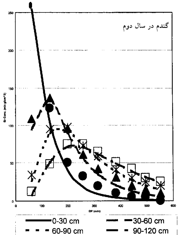
شکل ۲. غلظت‌های اندازه‌گیری شده (نشانه‌ها) و مقادیر برازش شده (خطوط) به وسیله مدل RSM در سال دوم. محور افقی نمودارها مقدار نفوذ عمقی (DP) بر حسب میلی‌متر و محور عمودی غلظت برماید بر حسب میکروگرم بر سانتی‌متر مکعب خاک است.
