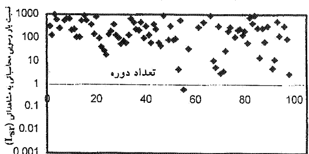
نمودار ۳-۱۰. روش فاضل، رودخانه کارون
