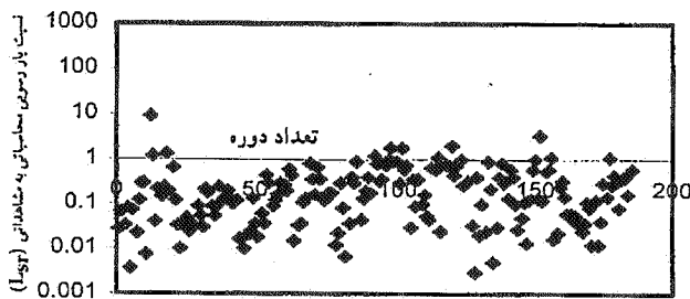
نمودار ۲-۹. روش بگ، رودخانه کرخه
