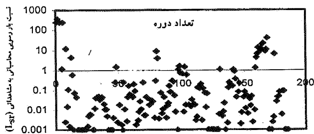
نمودار ۲-۸. روش یانگ، رودخانه کرخه
