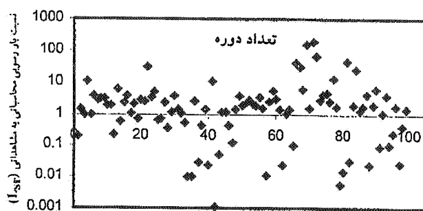
نمودار ۶-۲. روش وایف، رودخانه کرخه
