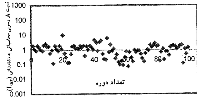
نمودار ۷-۳. روش انگلاند و هانسن، رودخانه کارون
