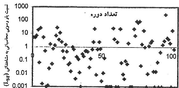
نمودار ۵-۱. روش وان ریجن، رودخانه دز
