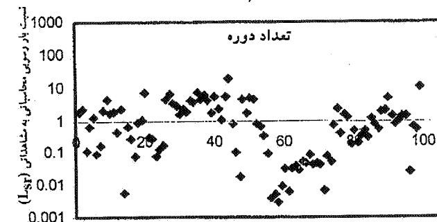
نمودار ۸-۳. روش یانگ، رودخانه کارون
