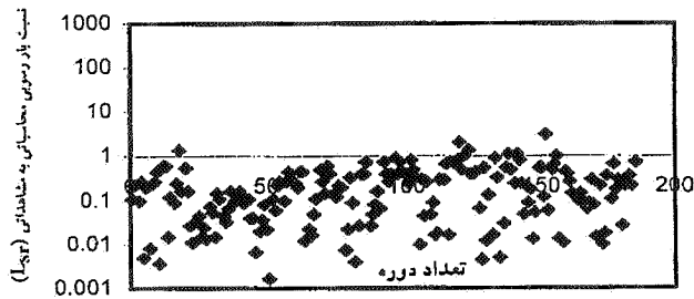
نمودار ۷-۲. روش انگلاند و هانسن، رودخانه کرخه
