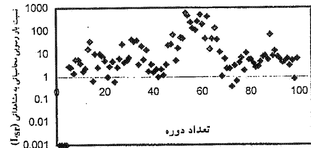
نمودار ۸-۱. روش یانگ، رودخانه دز
