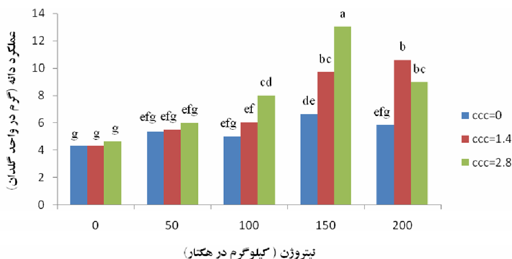
شکل ۱. میانگین عملکرد دانه در واحد گلدان تحت تأثیر نیتروژن و میزان CCC مصرفی. ستون‌هایی که دارای حروف مشترک هستند اختلاف معنی‌داری در سطح ۵٪ ندارند.
