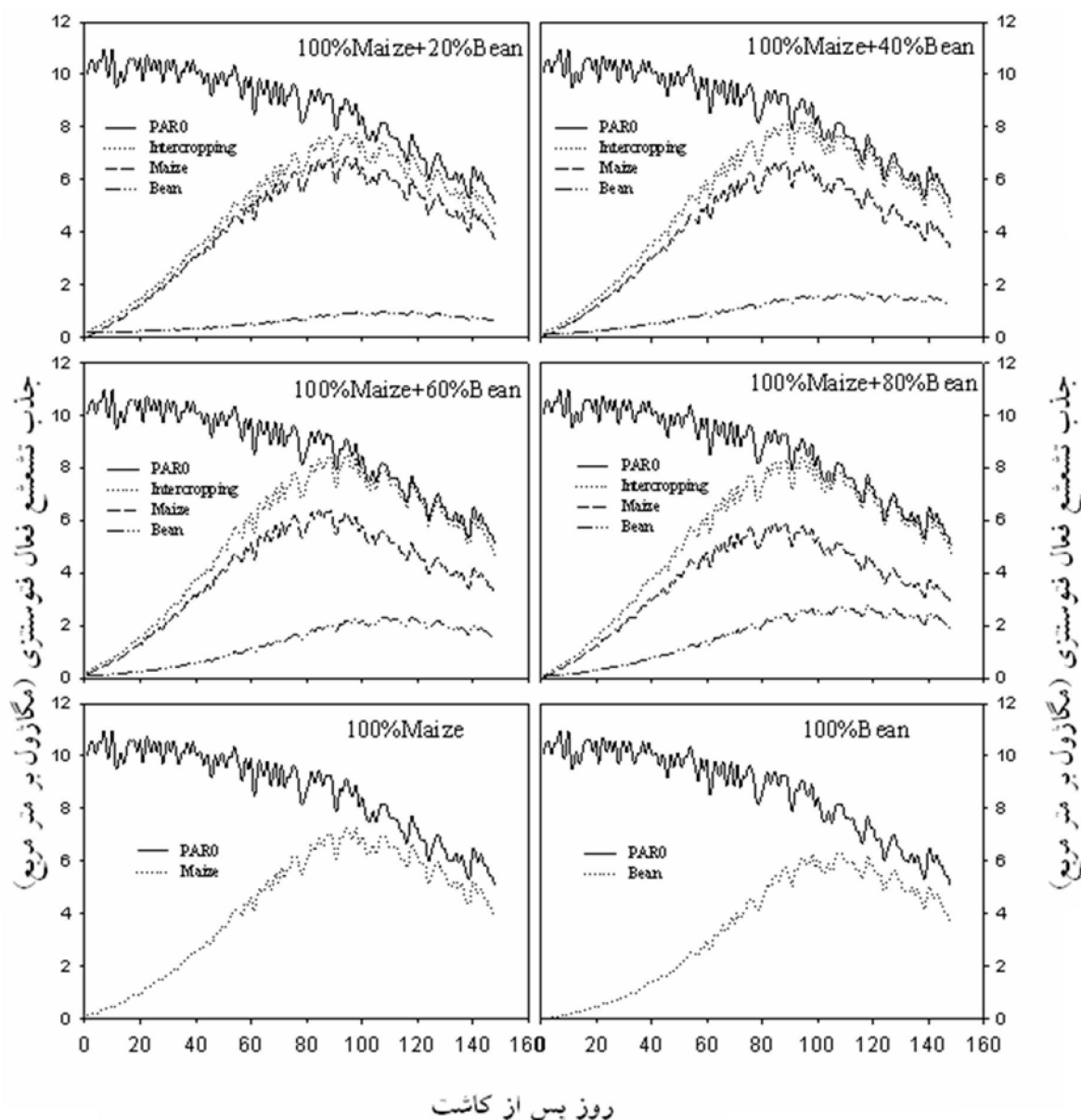
شکل ۲. روند تغییرات میزان تشعشع فعال فتوسنتزی رسیده به بالای سایه انداز (PAR0)، میزان تشعشع فعال فتوسنتزی جذب شده توسط سایه انداز مخلوط ذرت-لوبیا (Intercropping) و هم چنین سهم هر دو گیاه ذرت (Maize) و لوبیا (Bean) به صورت جداگانه در کشت مخلوط و خالص هر دو گونه
