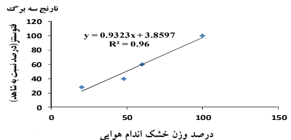
شکل ۳. همبستگی بین فتوستت با وزن خشک اندام هوایی در دو پایه بکرایی و نارنج سه برگ پس از ۸ هفته از
