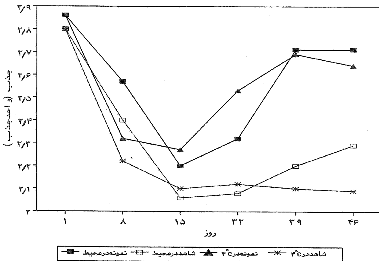
شکل ۶. مقایسه رنگ تولیدی (نمونه) و کارامل (شاهد) در نوشابه زمزم، در دمای محیط و ۴°C
