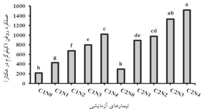
شکل ۲. مقایسه میانگین اثرات متقابل رقم \times مقدار کود نیتروژن در صفت عملکرد روغن کلزا طی دو سال زراعی C1 = رقم ساریگل C2 = رقم هایولا ۳۰۸ = N0 = شاهد (بدون مصرف کود نیتروژن) N1 = ۵۰ کیلوگرم در هکتار نیتروژن N2 = ۱۰۰ کیلوگرم در هکتار نیتروژن N3 = ۱۵۰ کیلوگرم در هکتار نیتروژن N4 = ۲۰۰ کیلوگرم در هکتار نیتروژن در هر ستون میانگین‌هایی که دارای حروف مشابه هستند، براساس آزمون دانکن در سطح احتمال پنج درصد تفاوت معنی‌داری ندارند.
