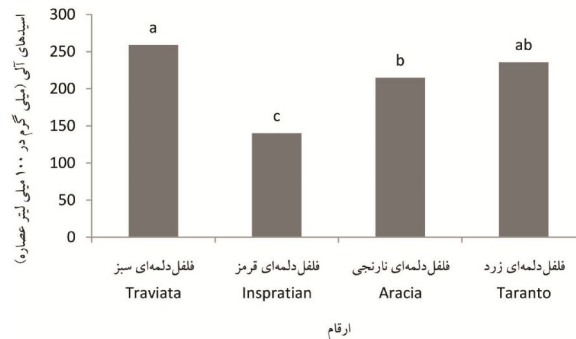
شکل ۲. مقایسه میانگین میزان اسیدهای آلی رقم های متفاوت فلفل دلمه ای. میانگین هایی که دارای حداقل یک حرف مشترک هستند در سطح احتمال ۵ درصد براساس آزمون LSD اختلاف معنی دار ندارند.
