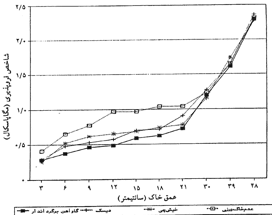
شکل ۲- روند تغییرات شاخص فروپذیری در اعماق مختلف خاک، در روشهای خاک‌ورزی تحت شرایط سوزاندن بقایای گیاهی در مرحله گلدهی
