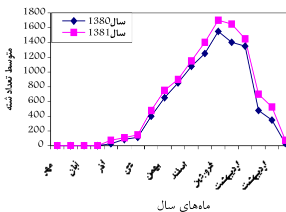
شکل ۱. متوسط تغییرات جمعیت شته در ایستگاه زهک در ۳۰ برگ
