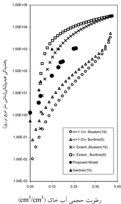
شکل ۲۱. پخشیدگی هیدرولیکی در خاک آرمود آغاچ (بافت لومی رسی شنی)
